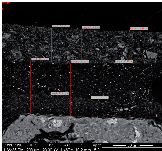
Figur 5: Malingslag på ny plade. Der ses umiddelbart 2 lag maling. Den nederste maling (den røde på figur 3), er dog lidt forskellig i struktur mellem top og bund, hvilket tyder på, at den er påført i to omgange. De små hvide korn i denne maling er jernpigment. Malingen på toppen indeholder relativt store pigmentkorn.
