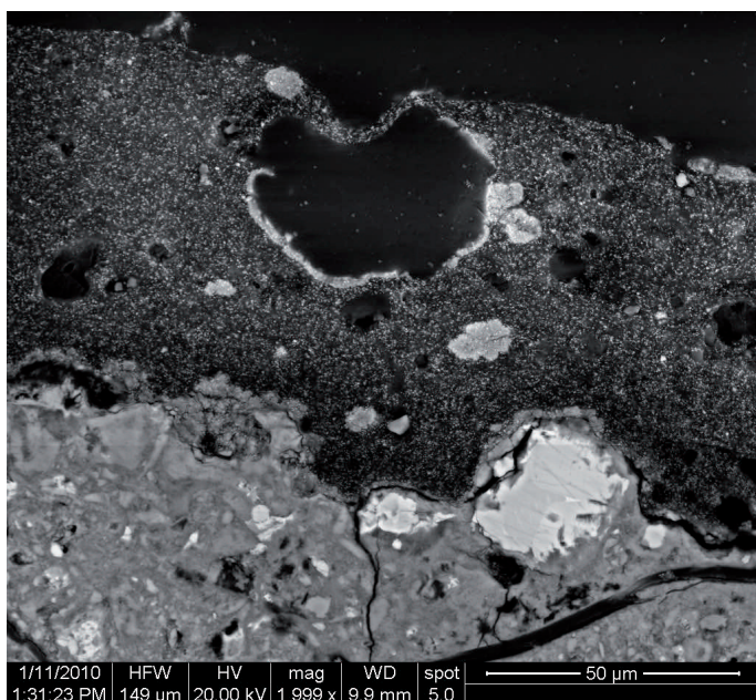
Figur 4: Malingslag på gammel plade. Der ses kun et lag maling; det brune materiale, som ses på det optiske billede (figur 2,) er grundet fiberbeton. Den grønne har en meget ensartet struktur bestående af små mineralske faser. De lyse udfældninger langs defekt i maling og på overflade (pile) er calcit.
