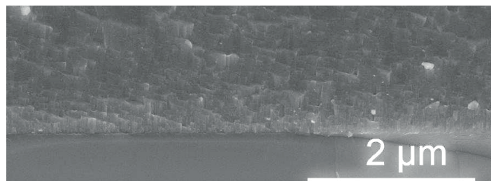
Elektronmikroskopibillede af et tværsnit af den finkornede TiBto-HP-belægning. Den meget tætte og finkornede struktur skyldes brugen af HiPIMS teknikken (se bagsiden).
