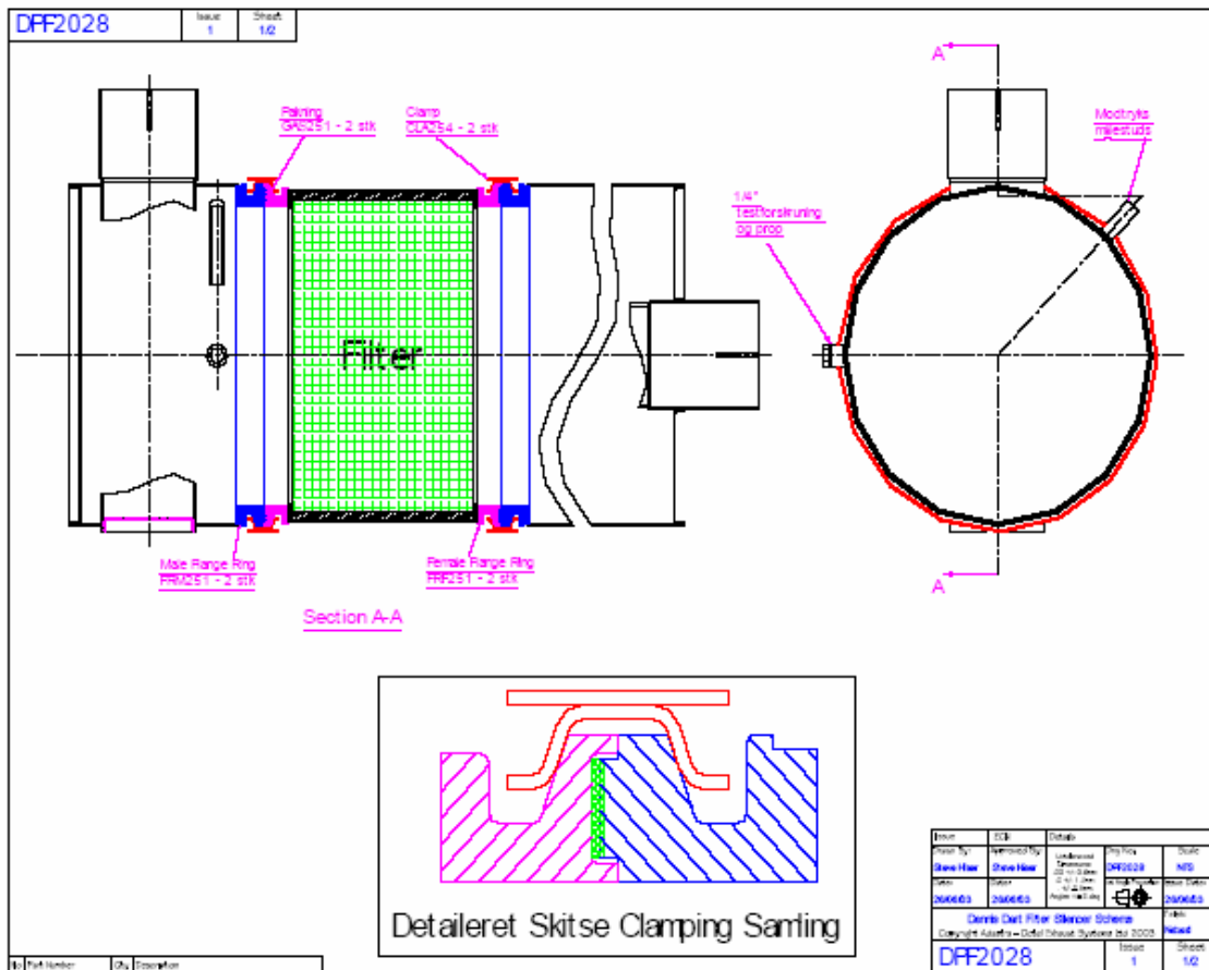
Fig 7. Typisk filter lyddæmper som viser clamps samlinger
