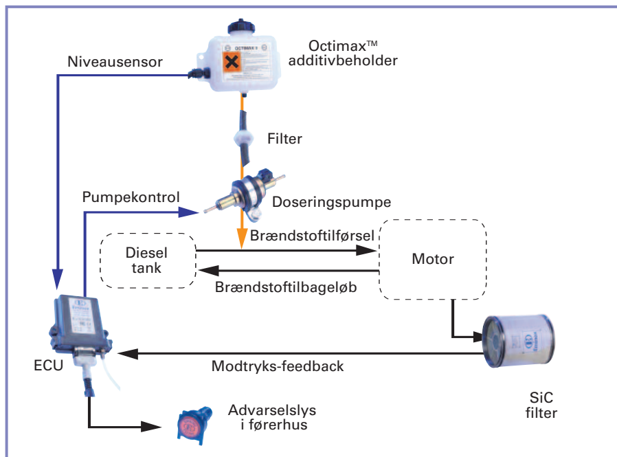
Figur 2 – Doseringssystem, skematisk installation
