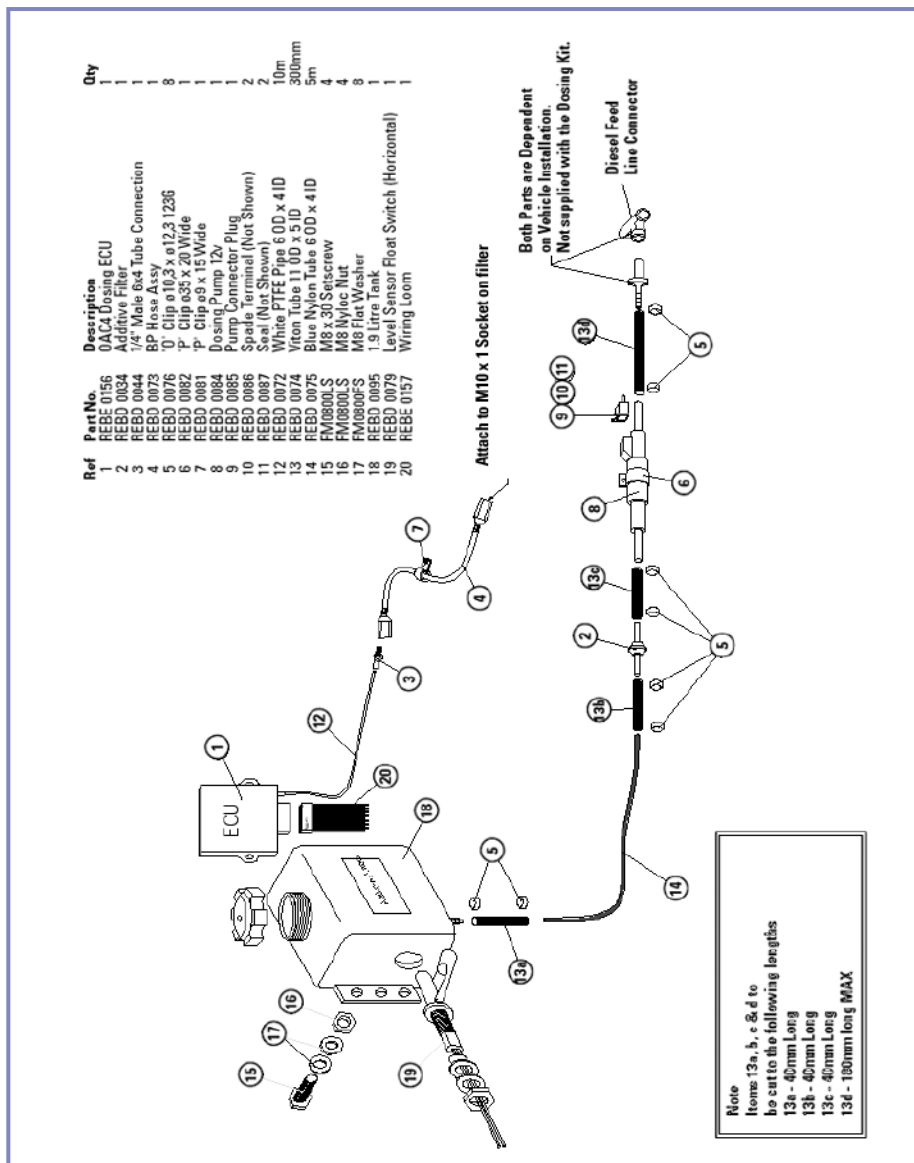
Figur 1 - detaljtegning af dele til FBC doseringssystemet
