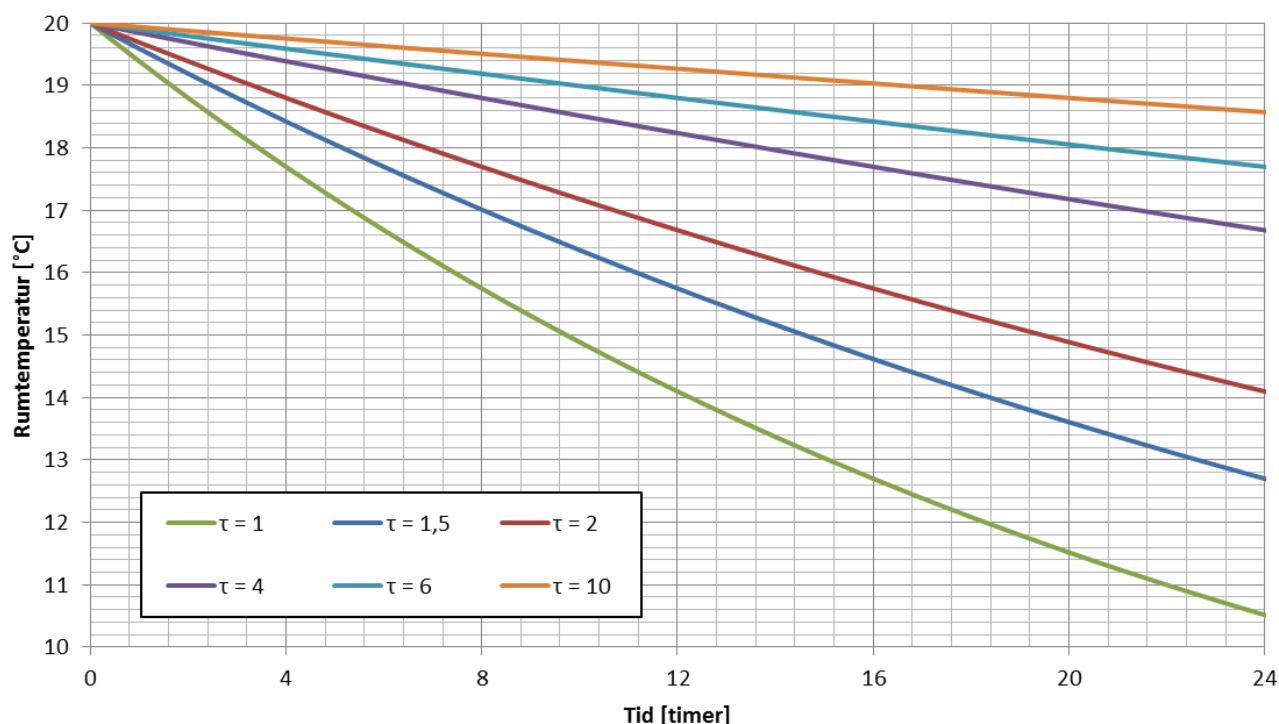
Figur 4.2: Illustration af forskellige tidskonstanter ( \tau ) udtrykt i døgn. Figuren viser rumtemperaturens fald fra en starttemperatur på 20 °C som funktion af tiden. Udetemperaturen er 5 °C.
