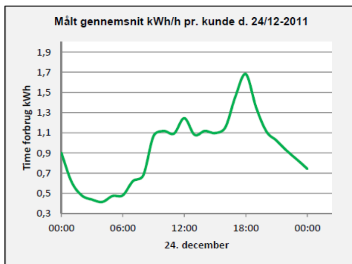
Figur 6.3: Målt belastningskurve på en udføring d. 24. december, der normalt er årets mest kritiske dato. Den karakteristiske spids omkring kl. 18 kaldes "kogespidsen" og året rundt ligger den dagligt hårdeste belastning omkring dette tidspunkt.
