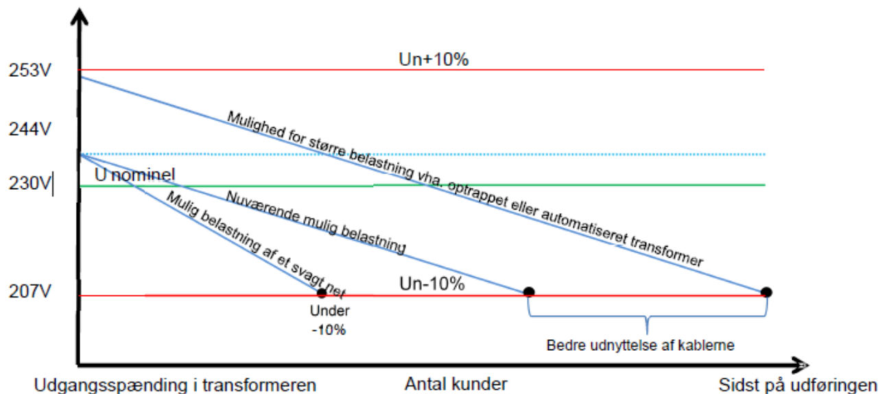
Figur 6.8: Illustration af belastninger ift. udgangsspænding fra transformere
