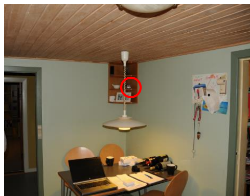
Fig. 10.4: Køkken. Rumføler i hjørneskab (DSC_6638)
