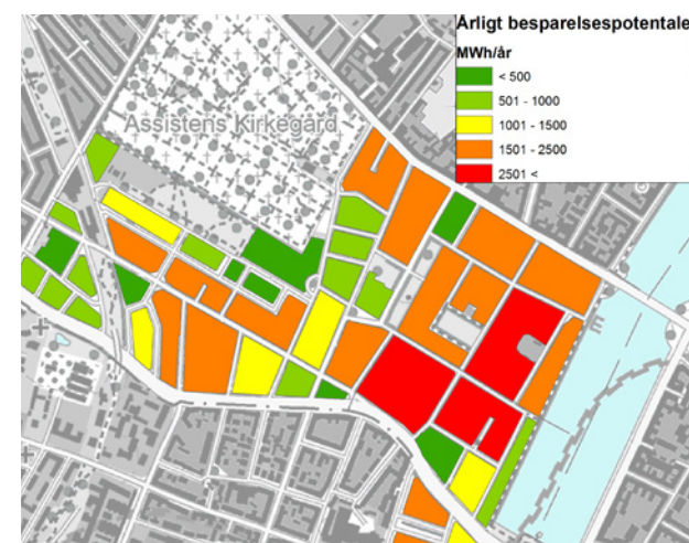
Figur 40. Eksempel på varmebesparelspotentiale på karreeniveau med 50% rumvarmebesparelse.
