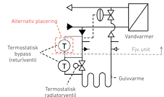
Figur 21. Brug af omløbsvand til opvarmning af badeværelsesgulv uden for opvarmningssæsonen.
