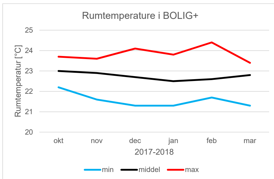
Figur 5.9 Minimum, middel og maksimum middelmåned rumtemperatur i BOLIG+ i opvarmningssæsonen 2017-2018.
