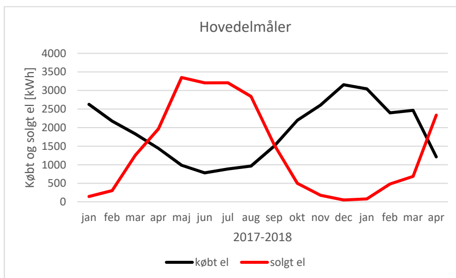
Figur 5.24 Købt og solgt el, målt med bygningens hovedelmåler.
