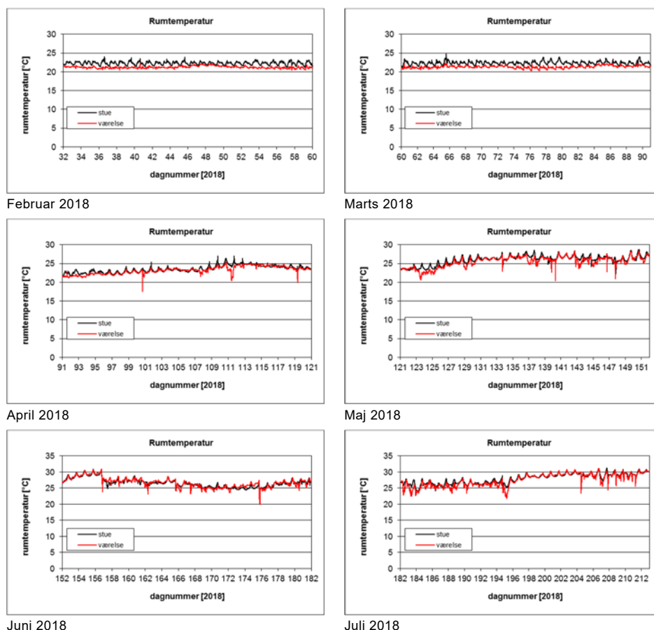
Figur 6.2 Rumtemperaturen i stuen og soveværelset gennem 16 måneder i én af lejlighederne i BOLIG+. Bemærk at y-aksen skifter fra maksimalt 30 °C til 35 °C for juni og juli 2018, da rumtemperaturerne her kommer over 30 °C.
