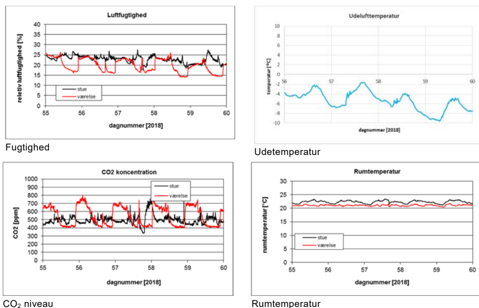
Figur 6.18 Relativ fugt, \text{CO}_2 og temperatur i soveværelset og stuen de fem dage sidst i februar 2018 i én af lejlighederne i BOLIG+.
