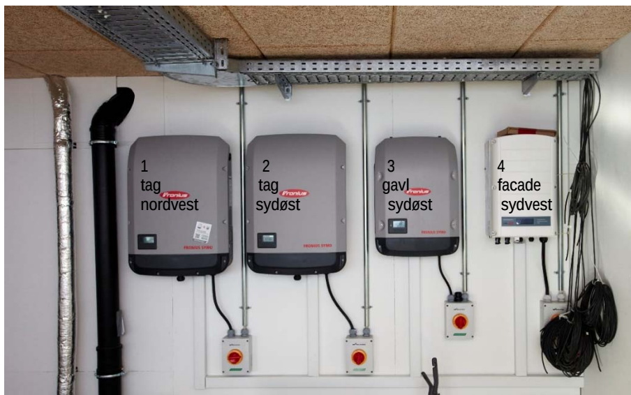
Figur 3.16 Solcelleanlæggenes fire invertere placeret i serviceetagen.
