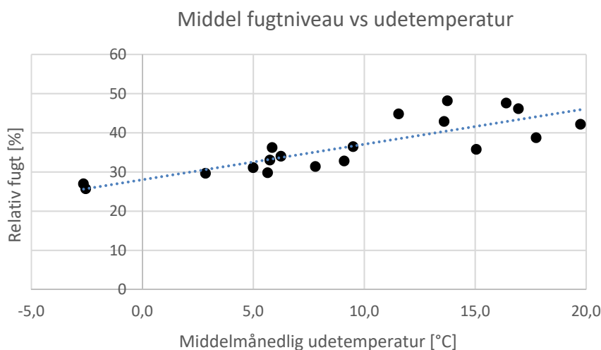
Figur 6.13 Månedsmiddel fugtniveau sammenlignet med middel månedlig udetemperatur.
