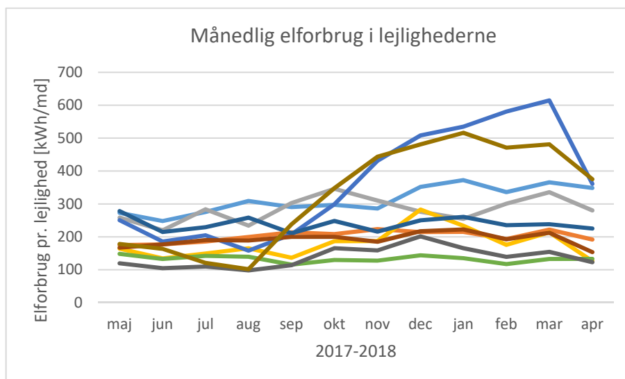
Figur 5.27 Lejlighedernes månedlige elforbrug.
