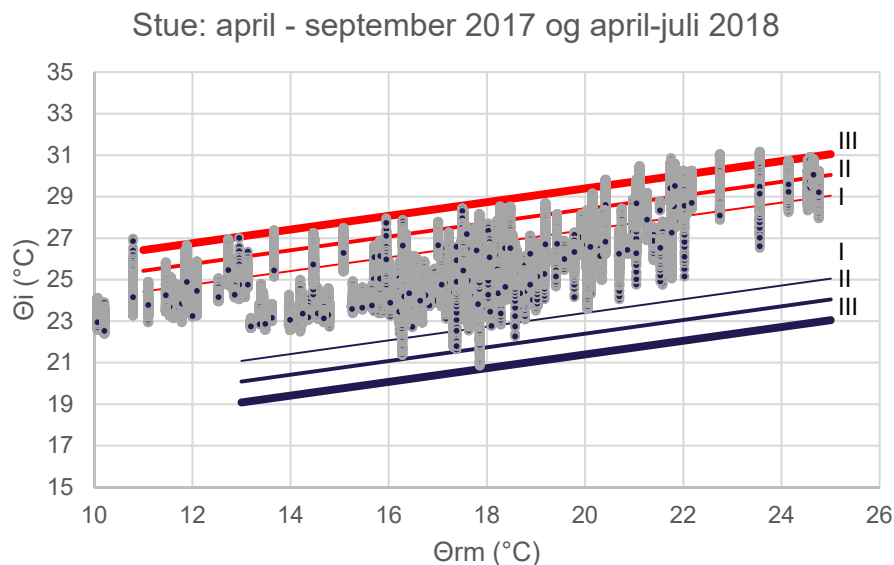
Figur 6.7 Eksempel på femminutters værdier af rumtemperaturen i stuen som funktion af den rullende middelværdi af udetemperaturen i én af lejlighederne. Værdierne er fra april-september 2017 og april-juli 2018.
