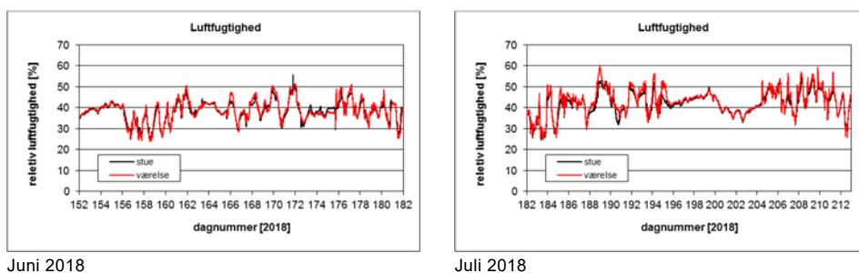
Figur 6.17 Relativ fugt i stuen og soveværelset gennem 16 måneder i én af lejlighederne i BOLIG+. Dog ikke i den, som skiller sig ud.
