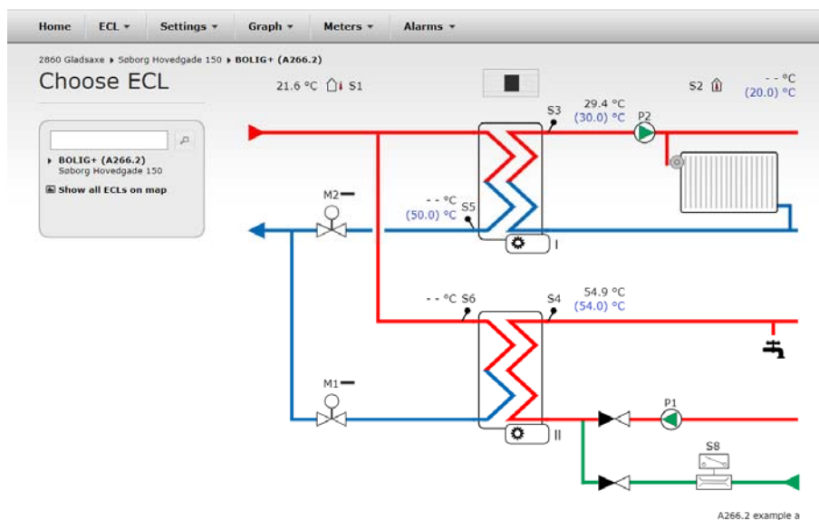
Figur 4.2 ECL 310 anvendes til styring af varmforsyningen i BOLIG+ Søborg (Danfoss).
