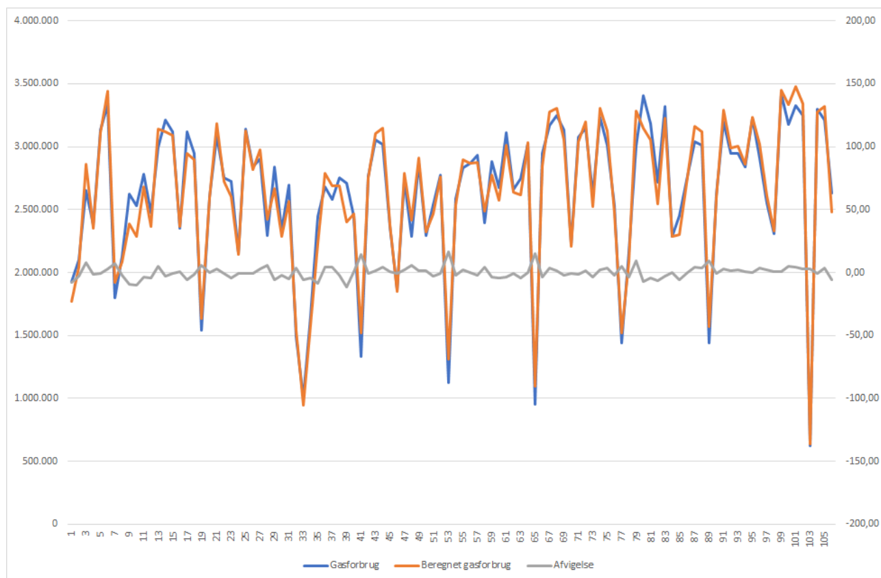
Figur 3.1.3 Beregnet og faktisk målt gasforbrug til ovnen.
