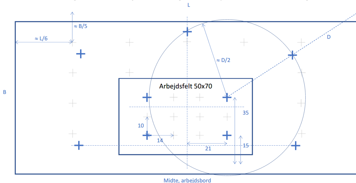
Figur 7.27. Målepunkter på arbejdsplads (arbejdsbord)
