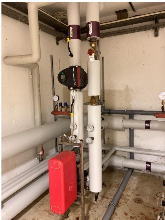
Figur 7.1. Fjernvarmeanlæg med veksler
