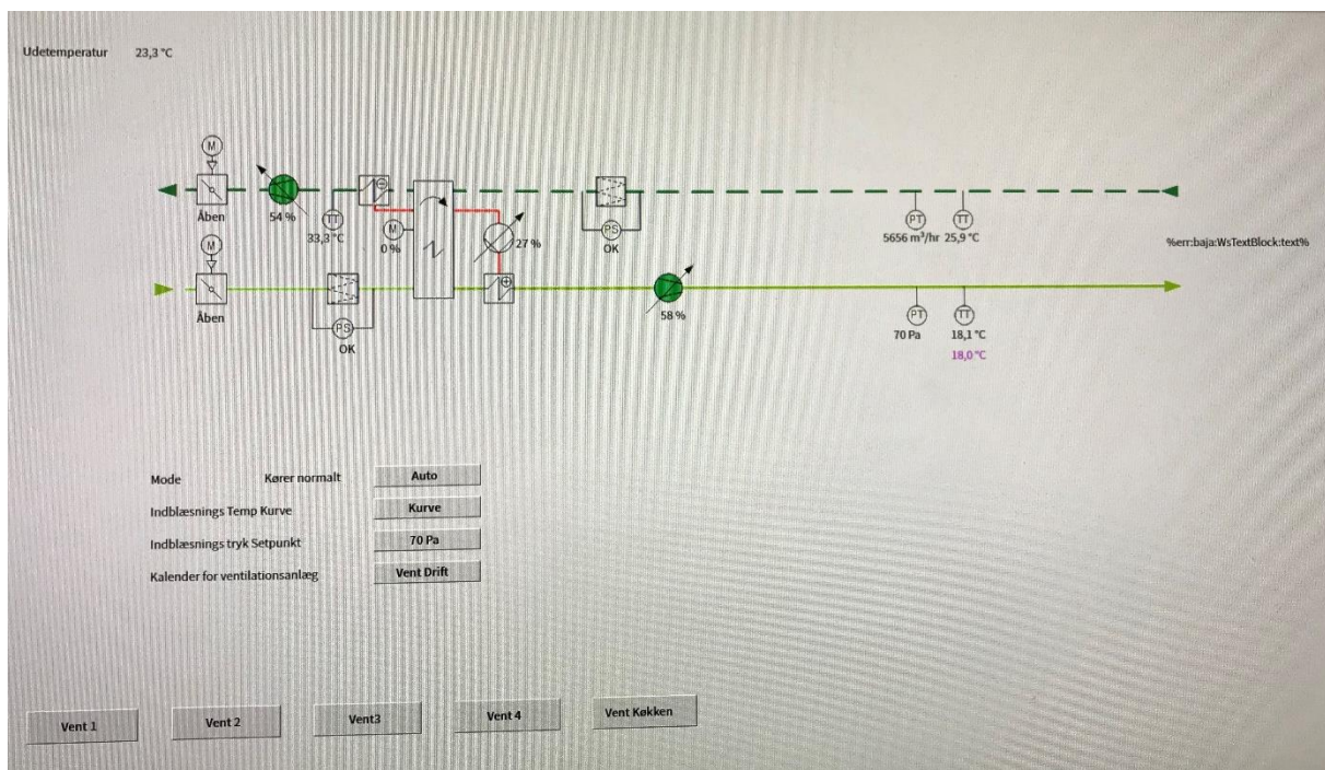
Figur 7.17. CTS-skærm. Ventilationsanlæg
