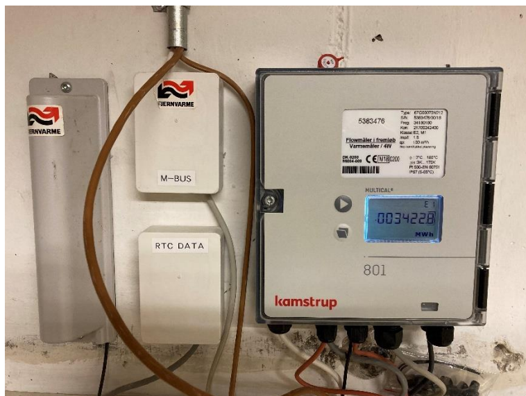
Figur 7.6 Vekslerens ydelse/effekt kan aflæses på varmemåleren, der desuden måler flow samt fremløbs- og returtemperatur
