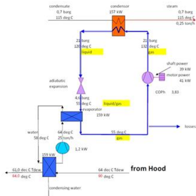
Figur 6.24 Prototypewarmepumpe fra IBK (NL) til produktion af damp ved ca. 115 °C baseret på R600 (butan) installeret ved papirfabrik [23].
