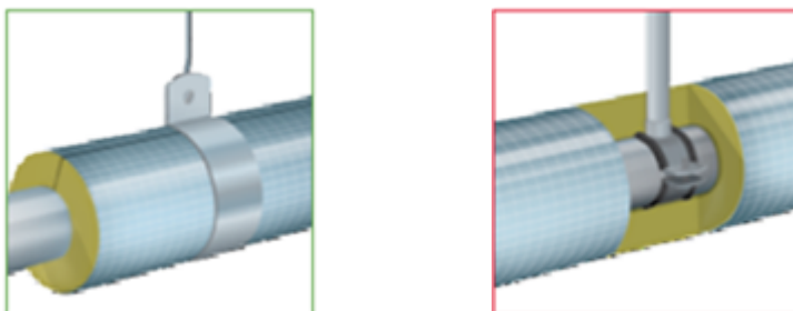
Figur 4.6 Venstre: Bæringer, der holder røret med halsjern uden på isoleringen. Højre: Bæringer, der holder røret med halsjern omkring røret, så bæringen gennembryder isoleringen.
