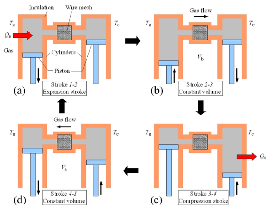
Figur 6.18 De fire delprocesser i varmepumpen efter Stirling-processen.
