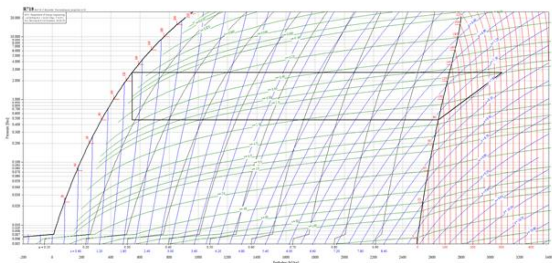
Figur 5.25 Eksemplet viser kredsprocessen for vand med fordampningstemperatur på 80 °C og kondensering 130 °C.
