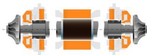
Figur 6.27 Totrinsdampkompressor baseret på JCI's turbochiller unit med magnetiske lejer. Billede fra testopstilling [25].
