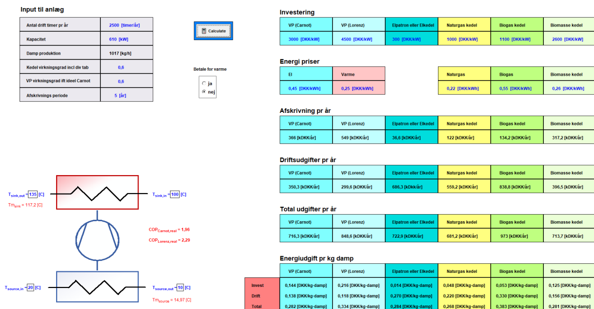
Figur 7.12 Eksempel på estimering af den forventede pris pr. produceret kg damp for forskellige energikilder (EES-model).
