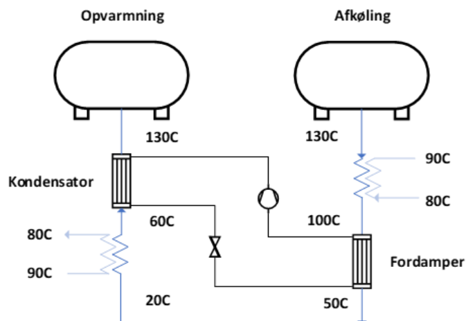
Figur 9.7 Skitse af installation af decentral varmepumpe til afkøling og opvarmning.
