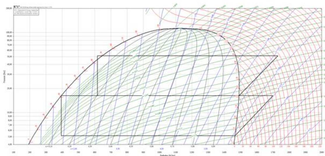
Figur 5.21 Et eksempel på et tottrins- \text{NH}_3 -anlæg med åben mellemkøler [17].
