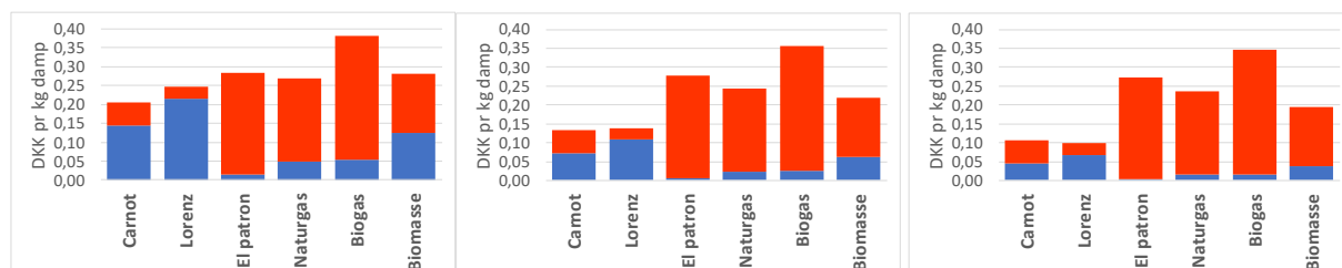
Figur 7.15 Eks.1 til Eks. 3 – udgifter til dampproduktion. Afkøling af varmekilden fra 100 °C til 80 °C og dampproduktion ved opvarmning fra 100 °C til 135 °C. Afskrivningsperiode på fem år og antal driftstimer hhv. 2500, 5000 og 8000 pr. år. Blå er investering, rød er driftsudgifter.
