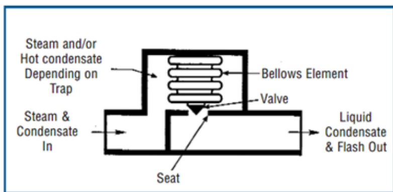
Figur 4.2 Bælgvandudlader [5].
