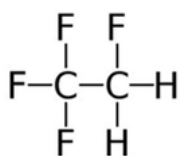
Figur 5.14 Et eksempel på HFC-kølemiddel, her R134a.
