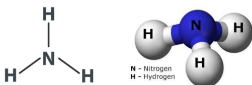
Figur 5.20 Den kemiske opbygning af ammoniak, \text{NH}_3 .
