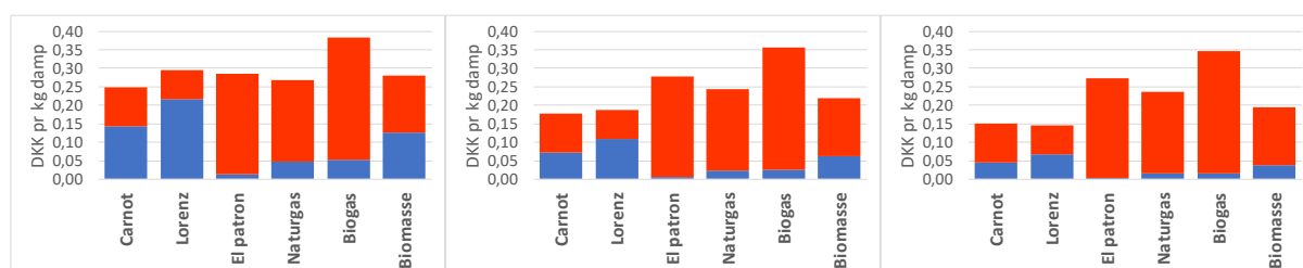
Figur 7.16 Eks. 4 til Eks. 6 – udgifter til dampproduktion. Afkøling af varmekilden fra 60 °C til 40 °C og dampproduktion ved opvarmning fra 100 °C til 135 °C. Afskrivningsperiode på fem år og antal driftstimer hhv. 2500, 5000 og 8000 pr. år.
