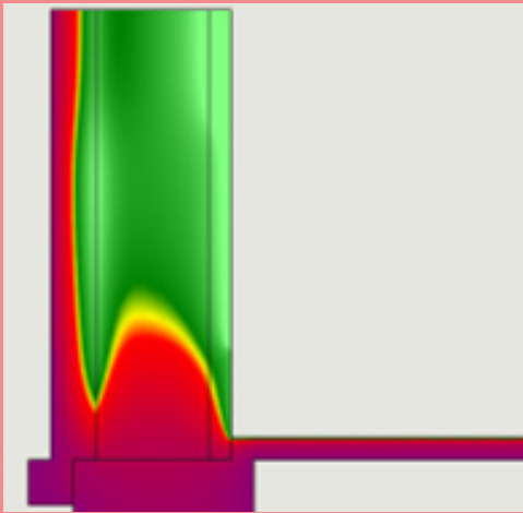
Diffusionsåben isolering
