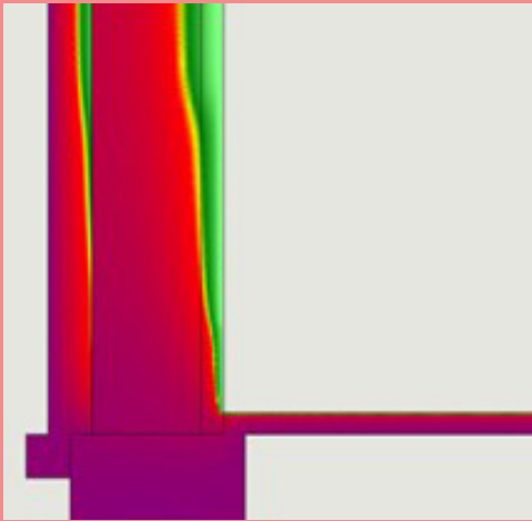
EPS-isolering + grundmursplade
